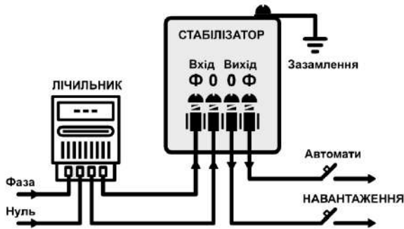
Рис.7 – Схема підключення стабілізатора до однофазної мережі
