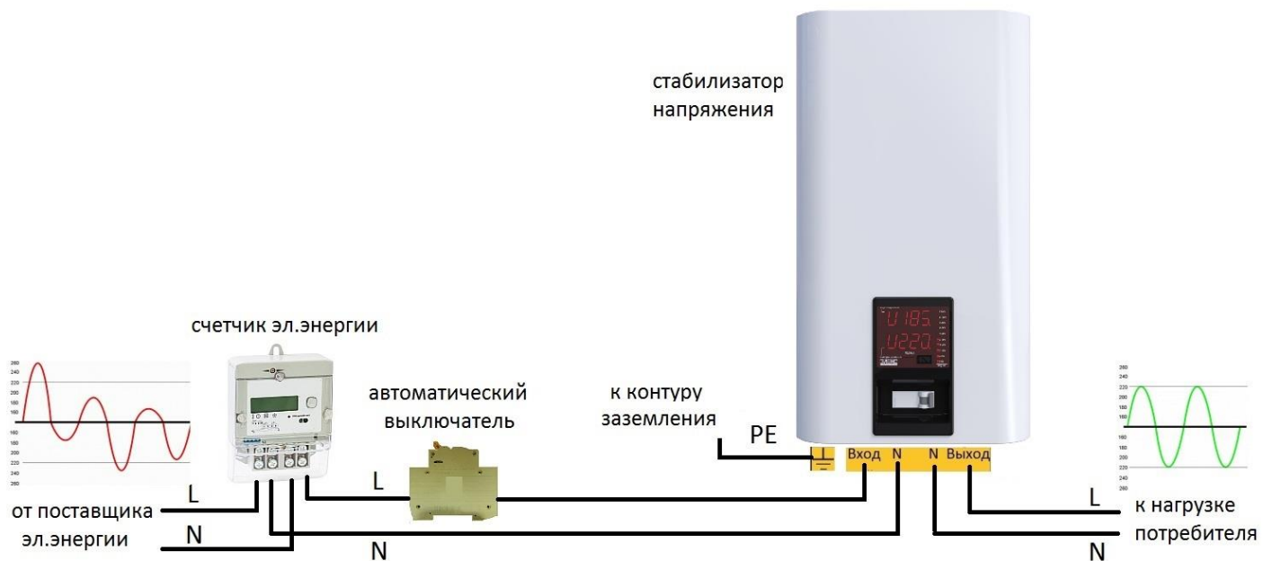
Рисунок 7. Схема подключения стабилизатора к однофазной сети
