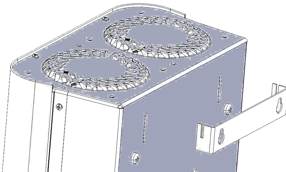
Рисунок 4. Крепление стабилизатора на установочную планку
