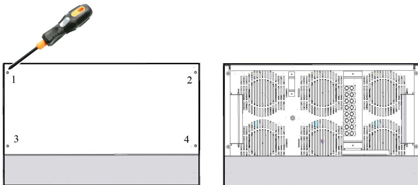
Рисунок 6. Схема снятия защитной крышки снизу корпуса стабилизатора
