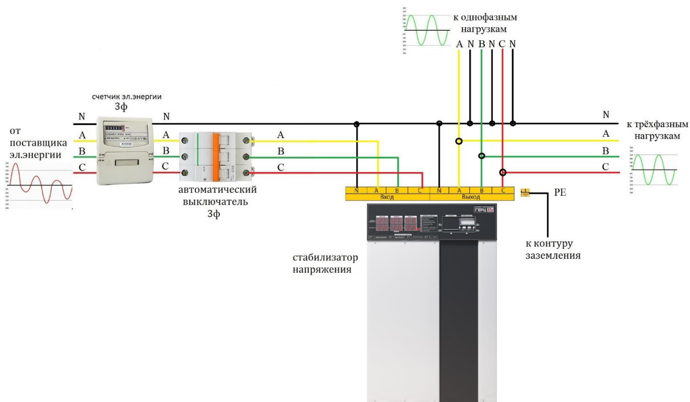
Рисунок 5. Схема подключения стабилизатора к трёхфазной сети
