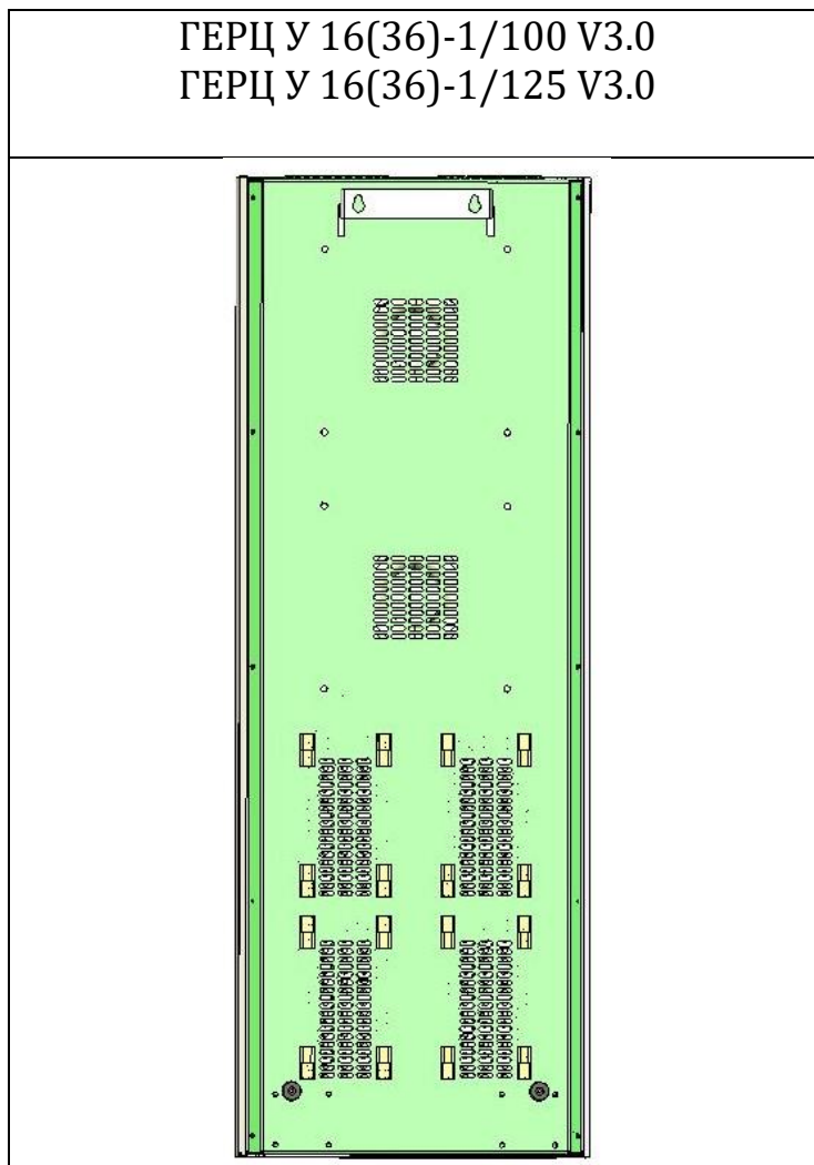
Рисунок 6. Установчі розміри стабілізаторів Герц на 100-125А
