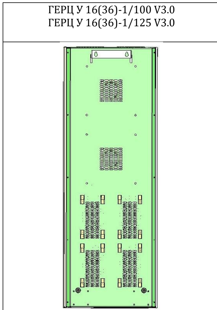
Рисунок 6. Установочные размеры стабилизаторов Герц на 100-125 А
