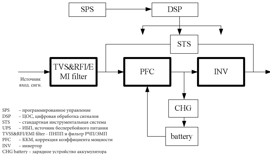
Рис. 1-3. Система ИБП
