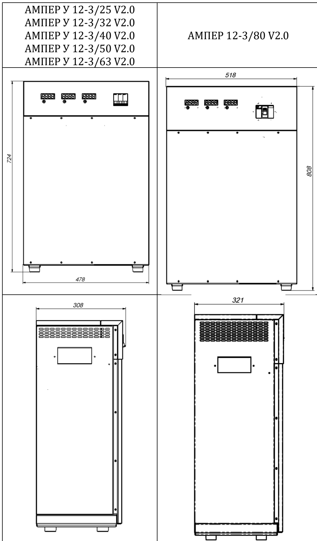
Рисунок 4. Габаритні розміри стабілізаторів
