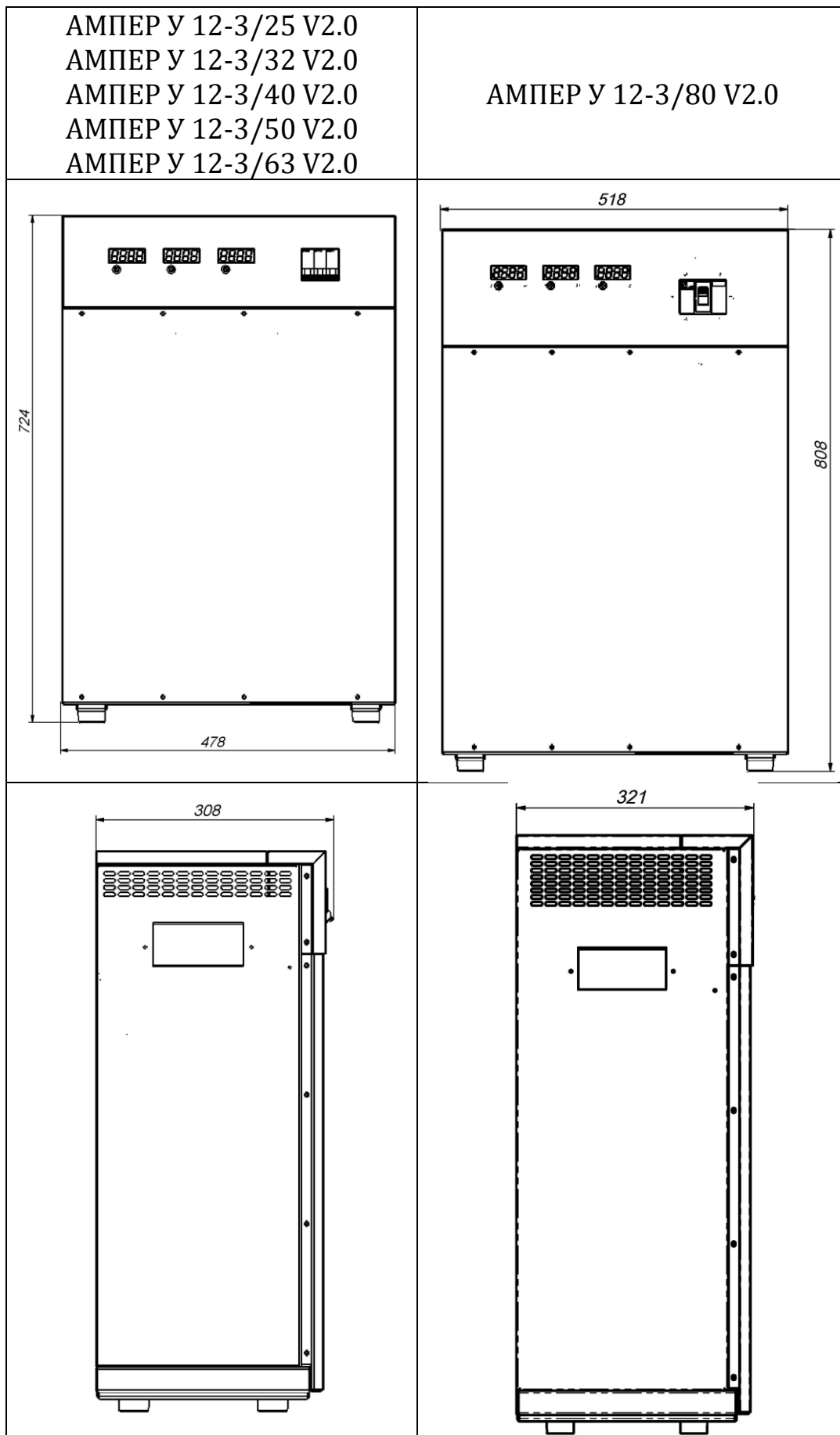
Рисунок 4. Габаритные размеры стабилизаторов
